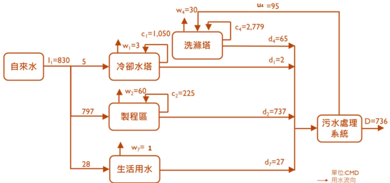
附圖 1 用水平衡圖繪製範例
