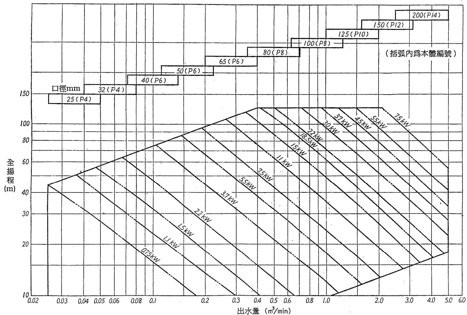
圖 6 性能圖表(50Hz)
