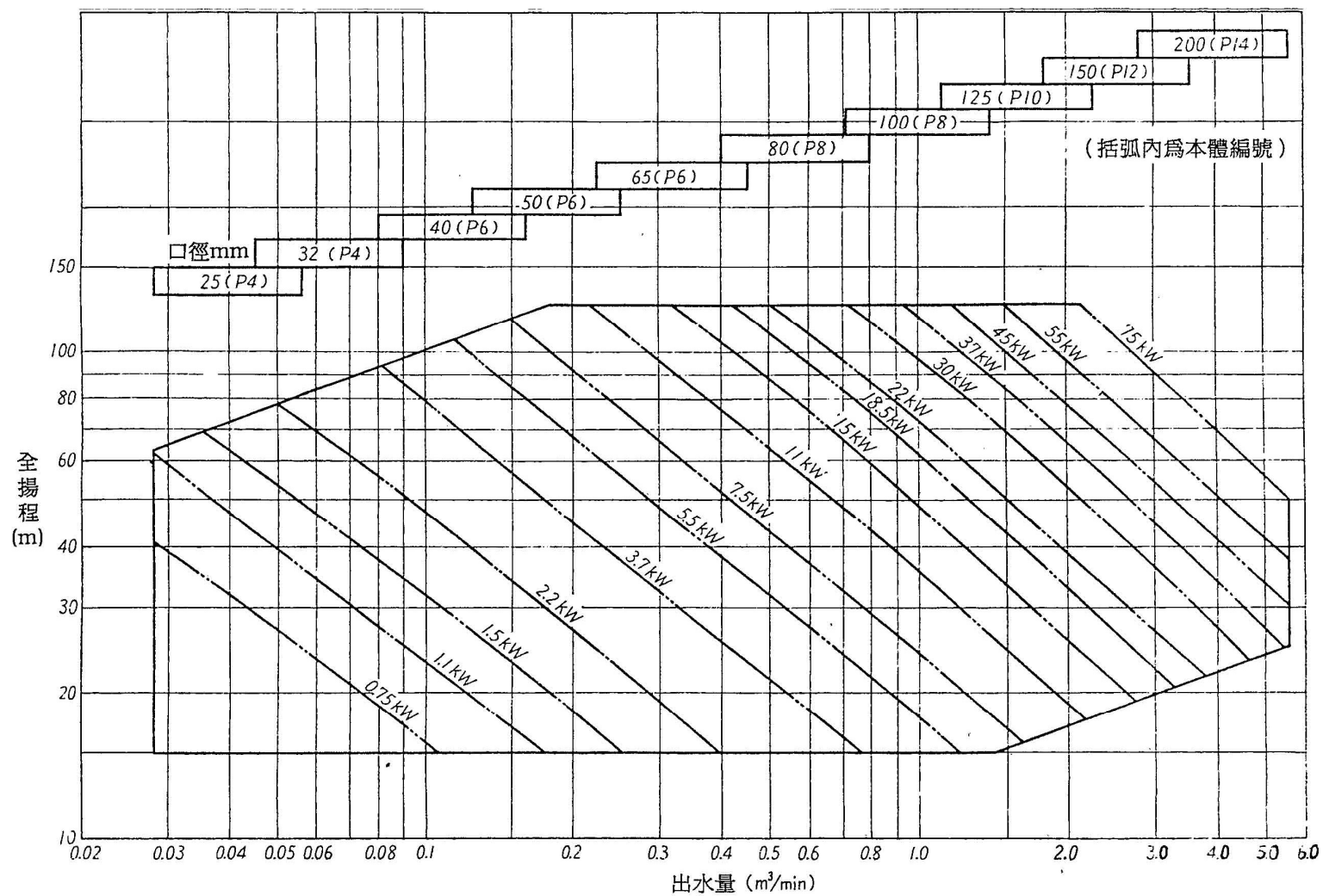
圖 7 性能圖表(60Hz)
